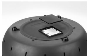
Fig1. Insira as 4 pilhas AA.
